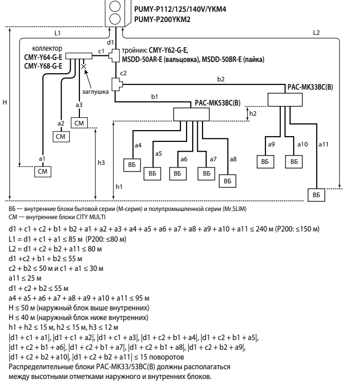
2 блока-распределителя
