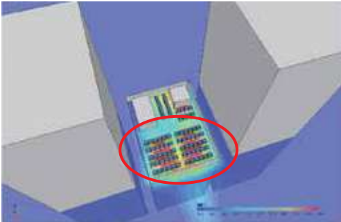
Групповая установка на кровле вблизи ограждений или при плотной застройке
