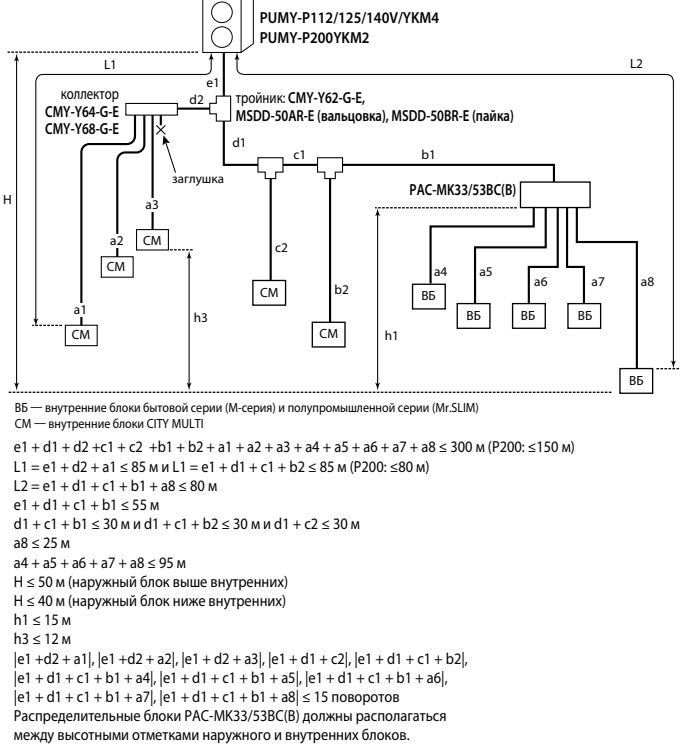
1 блок-распределитель
