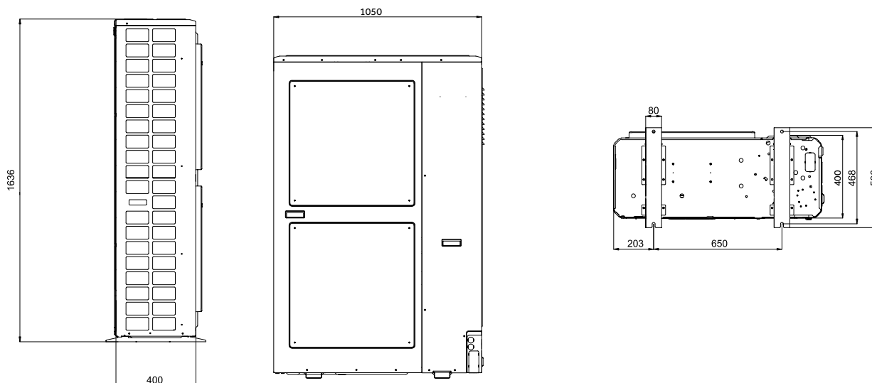
1UH200W1ERK, 1UH250W1ERK
